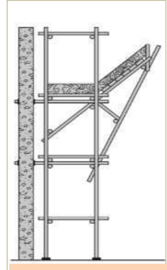
Figure33: Catchplatform/ fan
